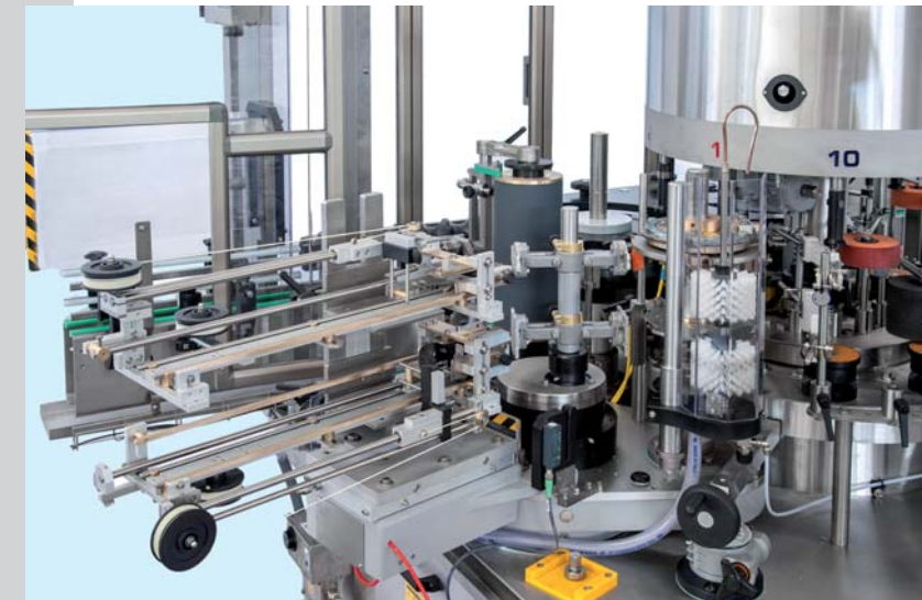
Stazione di etichettaggio tipo CG 84/A con sistema lavaggio pinze CG 84/A labeling station with pincer washing system Poste d'étiquetage mod. CG 84/A avec dispositif de nettoyage des pinces Estación de etiquetado tipo CG 84/A con sistema de lavado de pinza Etiketterstation Typ CG 84/A mit Reinigungssystem des Greiferzylinders
